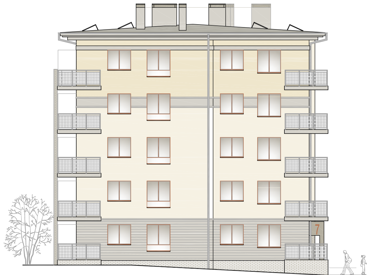
ELEWACJA PÓŁNOCNO - ZACHODNIA
